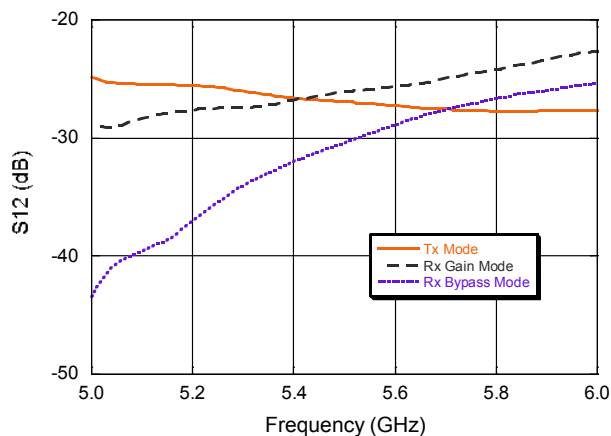
T_x - R_x Isolation
