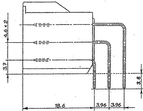
VERSIONE A 90°
