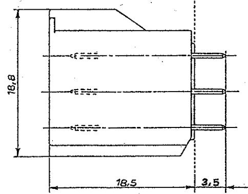
VERSIONE A 180°
